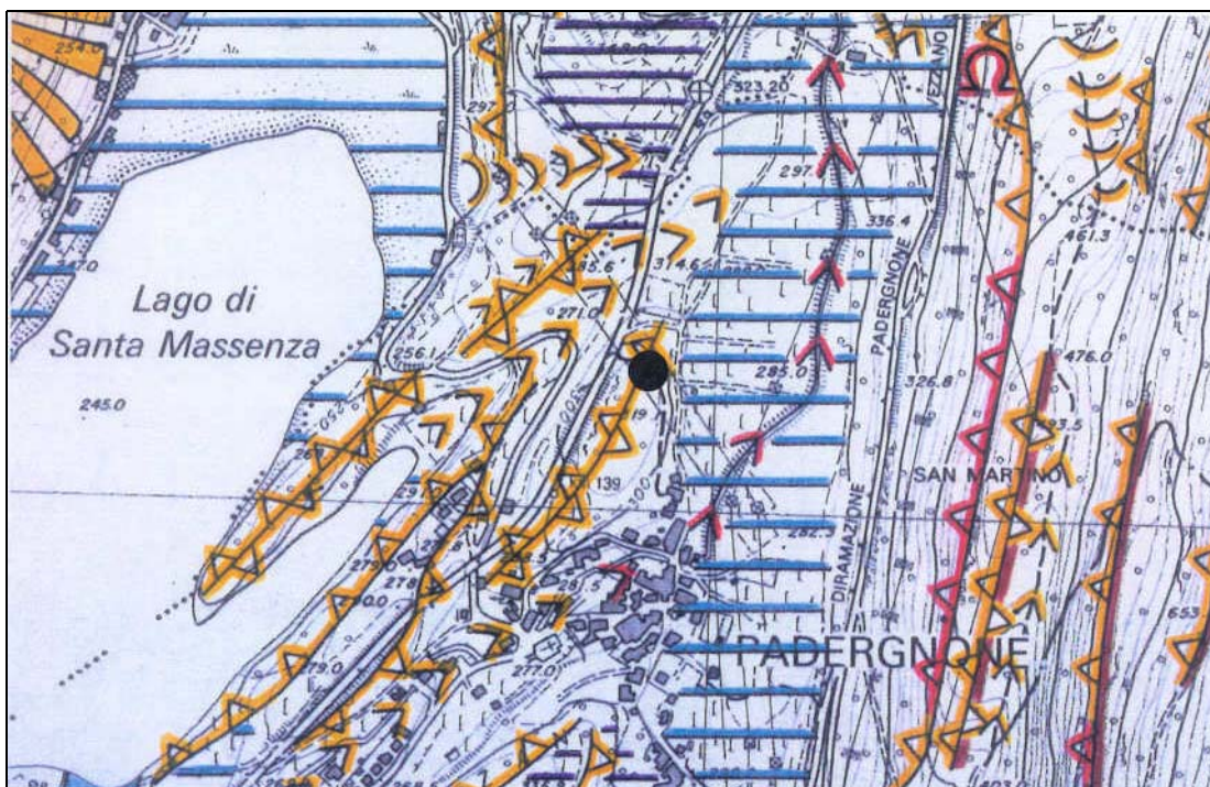
CARTA GEOMORFOLOGICA
