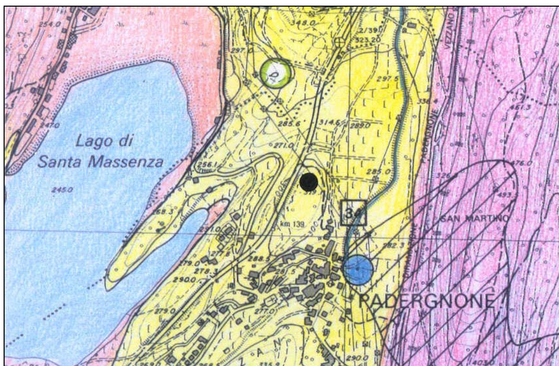
CARTA IDROGEOLOGICA
